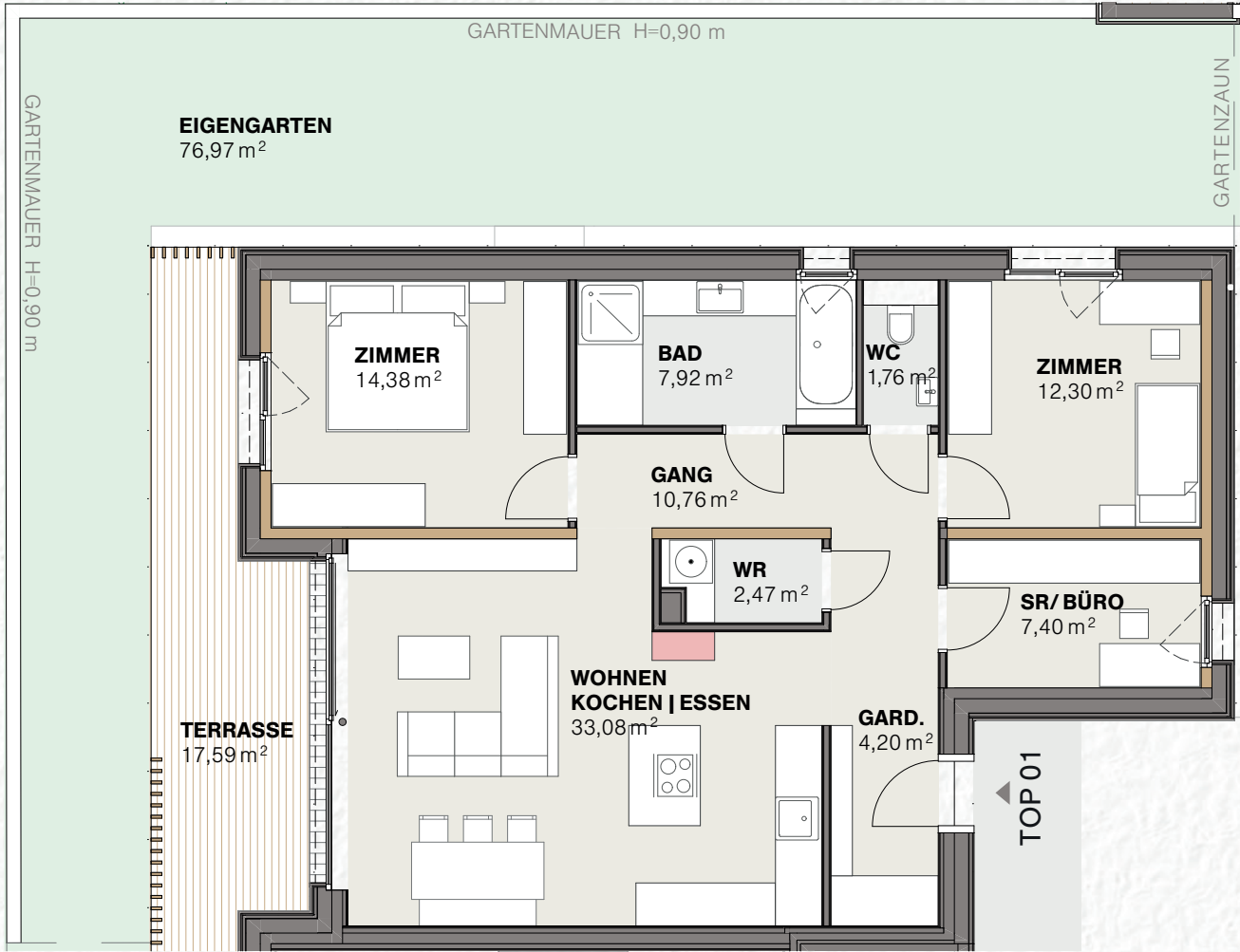
GRUNDRISS TOP 01 – 1:100
