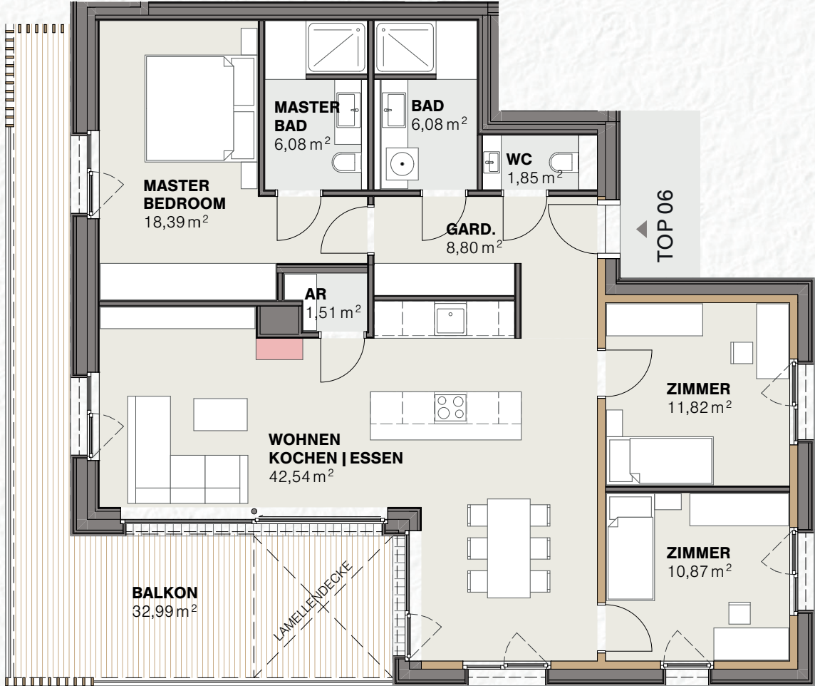
GRUNDRISS TOP 06 – 1:100
