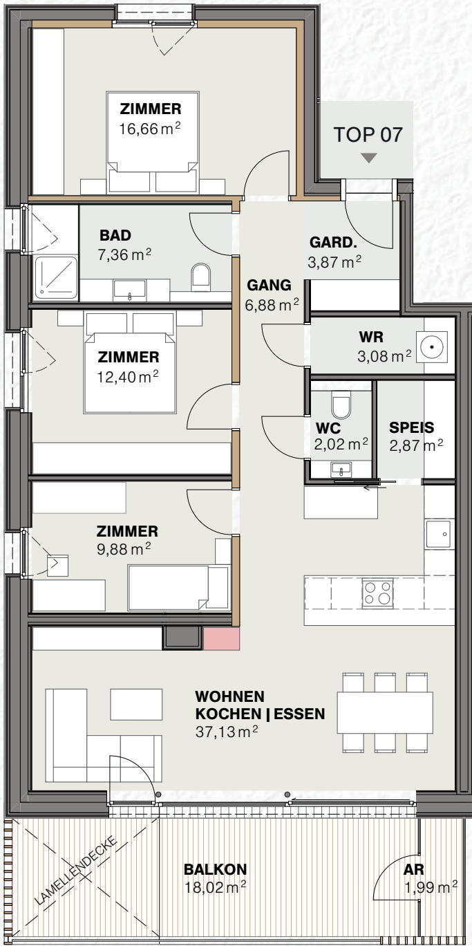
GRUNDRISS TOP 07 – 1:100
